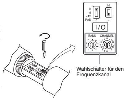
PAD-Schalter
